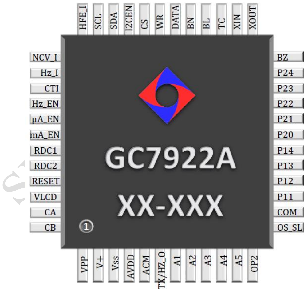
GC7922 LQFP48 封装管脚图
